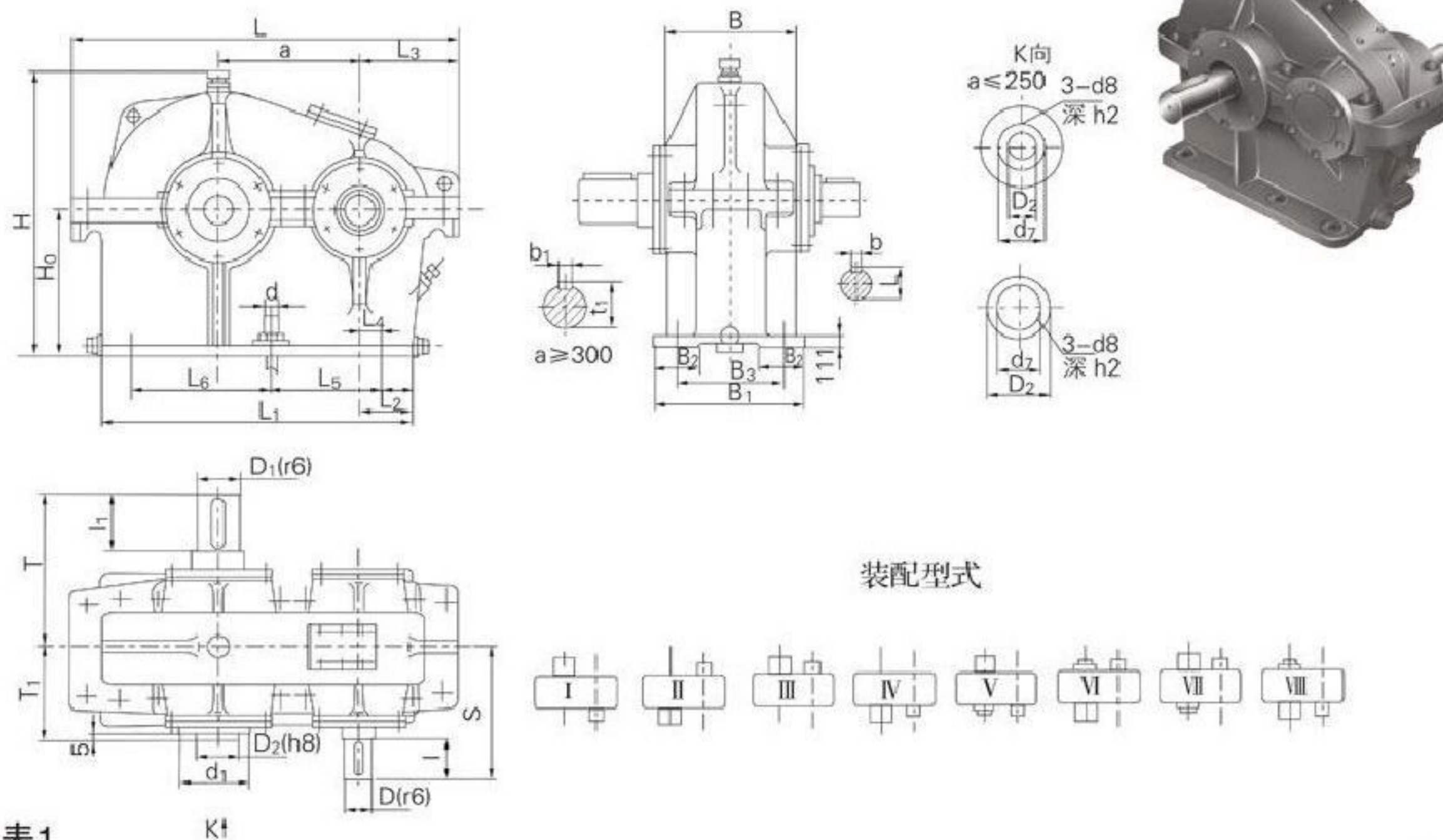
ZD 型减速机外形安装尺寸和装配型式
