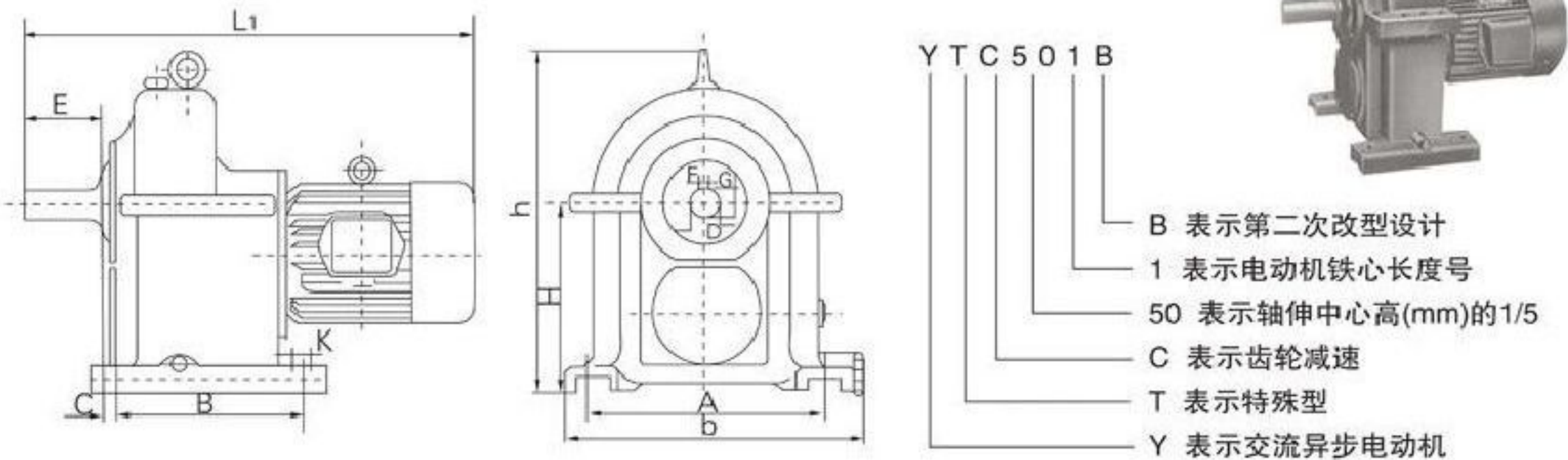
YTC型减速电机外形和安装尺寸
