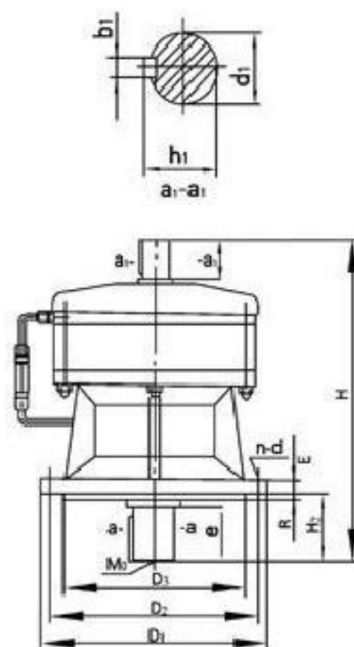
XL(BL)型
