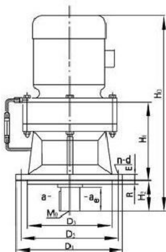
XLD(BLD)型
