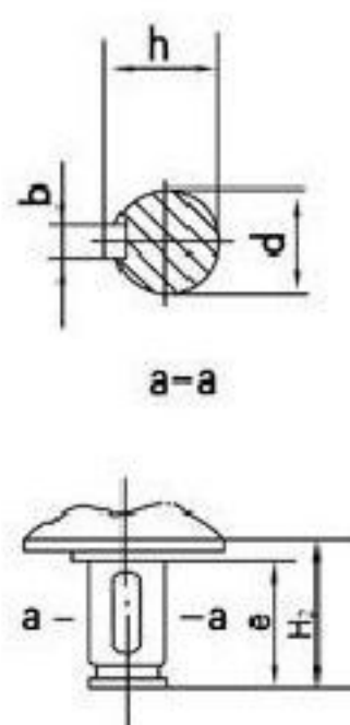
(夹壳型轴伸)
