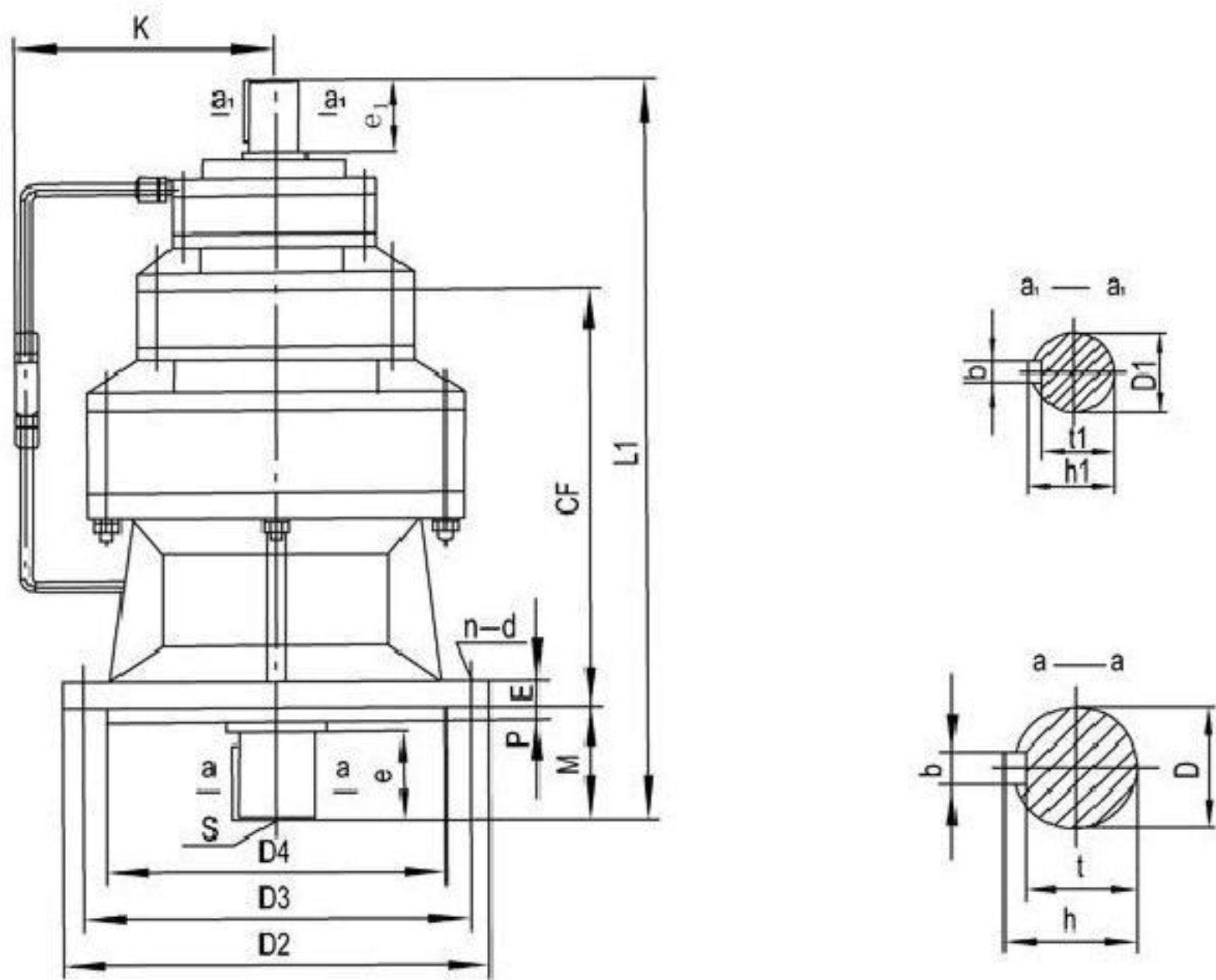
XLS型
