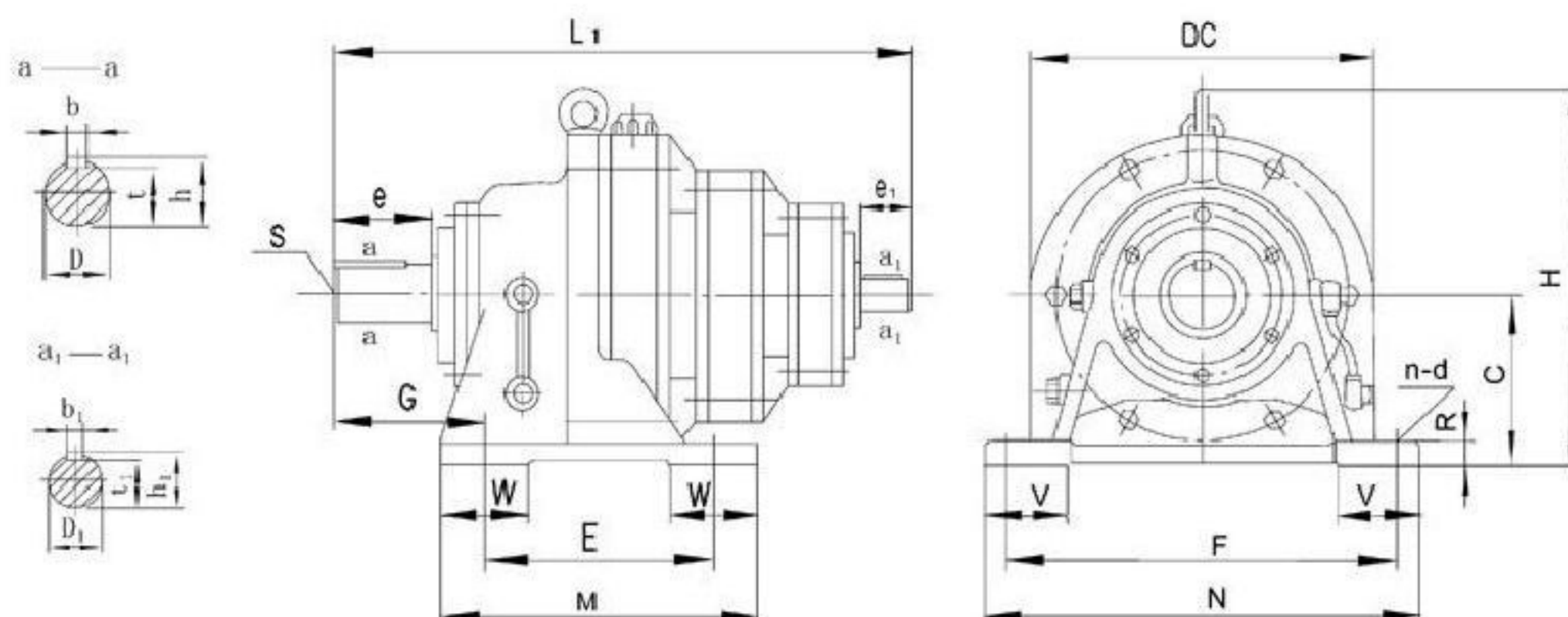
XWS型
