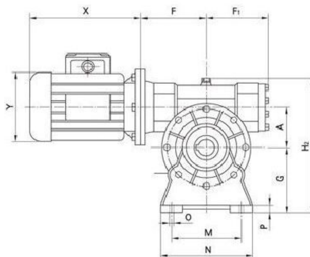
MWVF.../A
