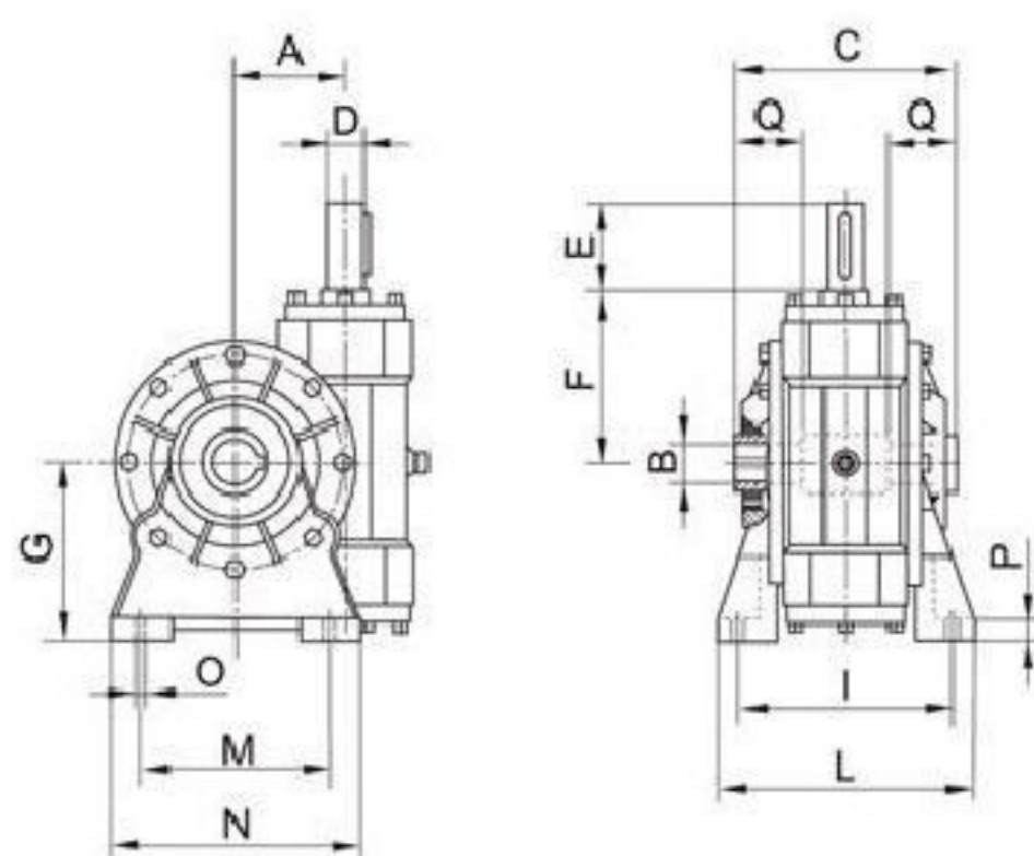
WVF.../V
