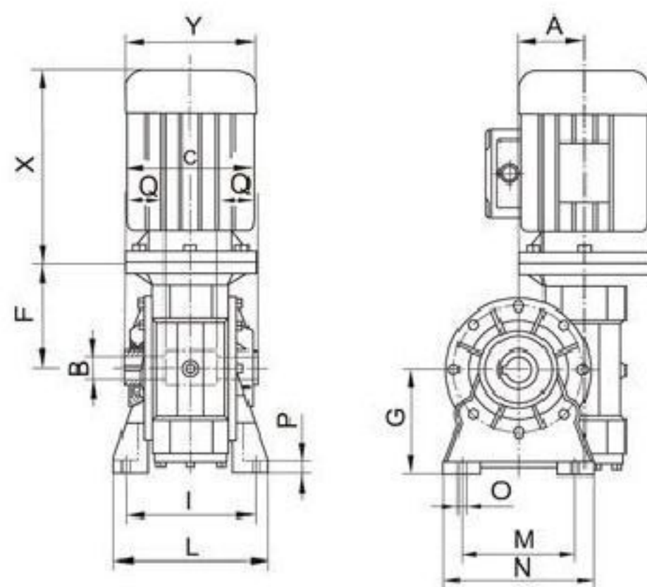
MWVF.../V
