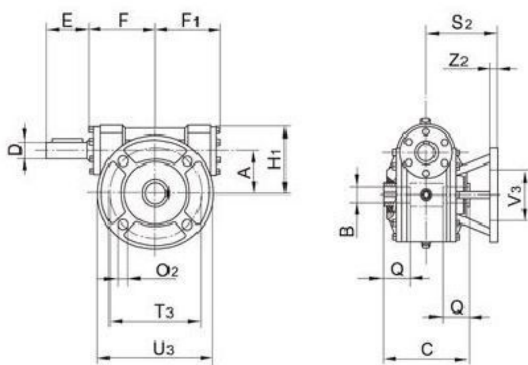
WVF.../FA
