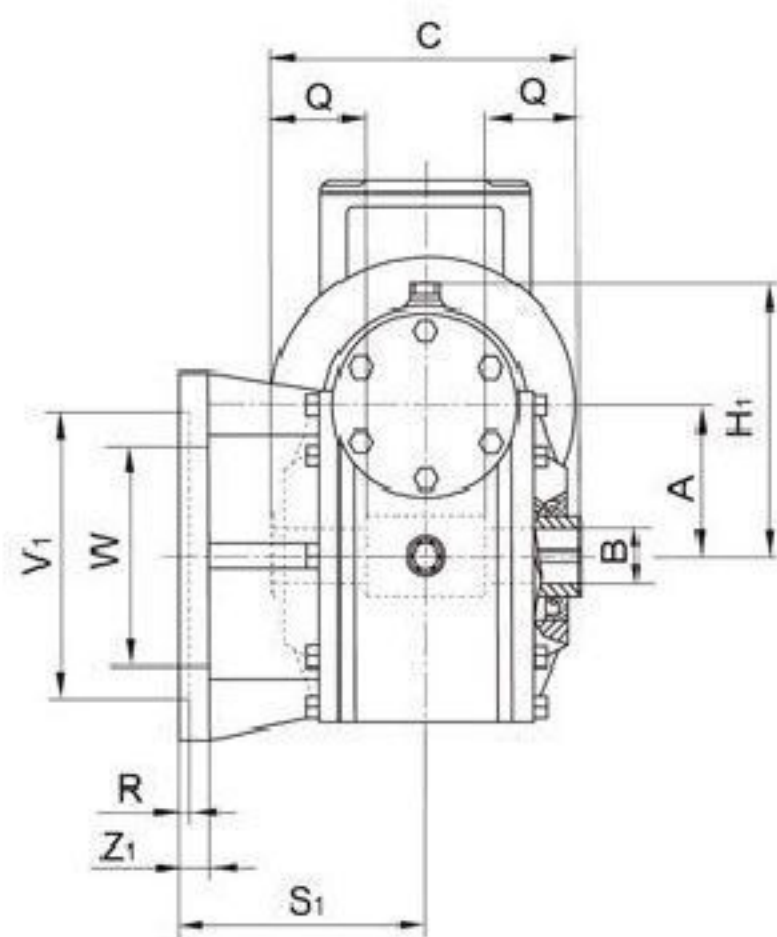
MWVF...FC -FR
