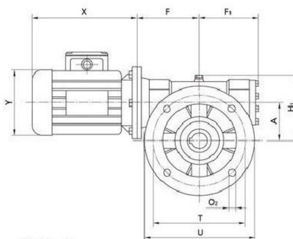
MWVF.../F
