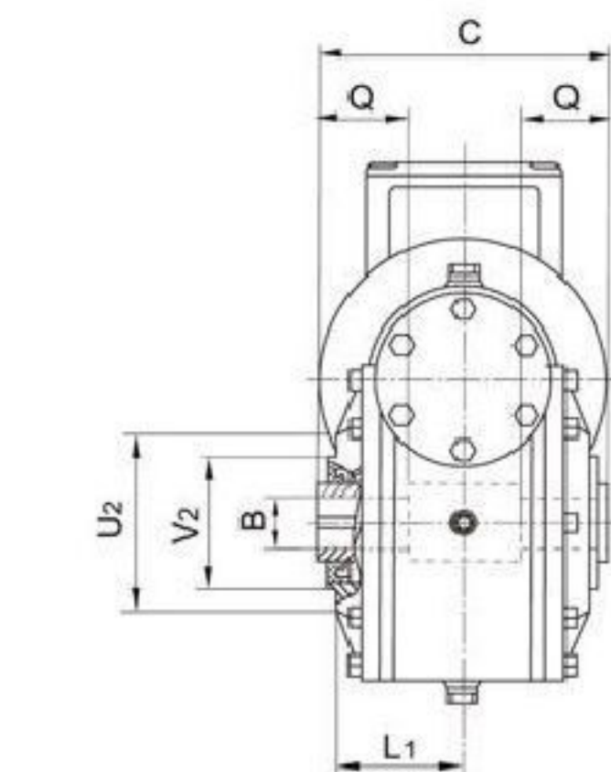
MWVF.../P
