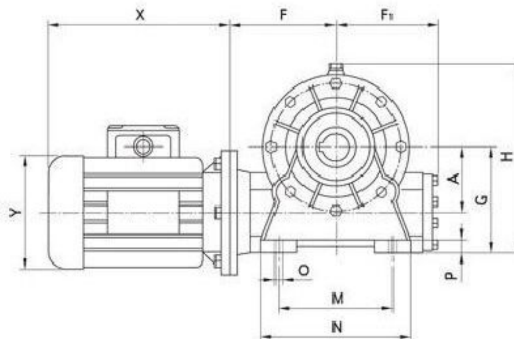
MWVF.../N
