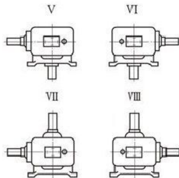
装配形式
