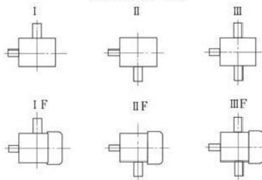
装配型式(K向)
