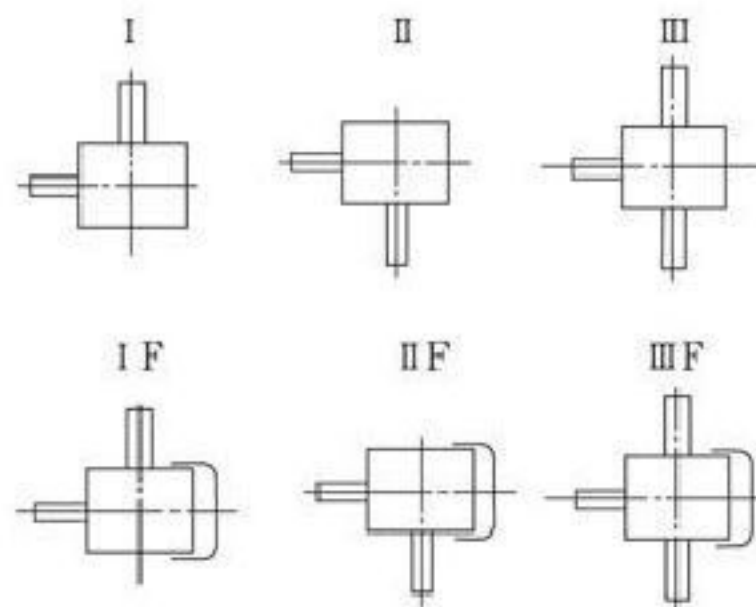
装配型式（K向）
