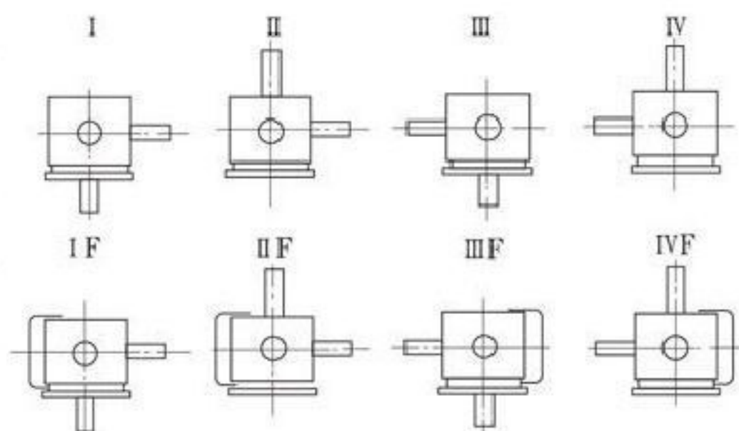
装配型式(K向旋转)
