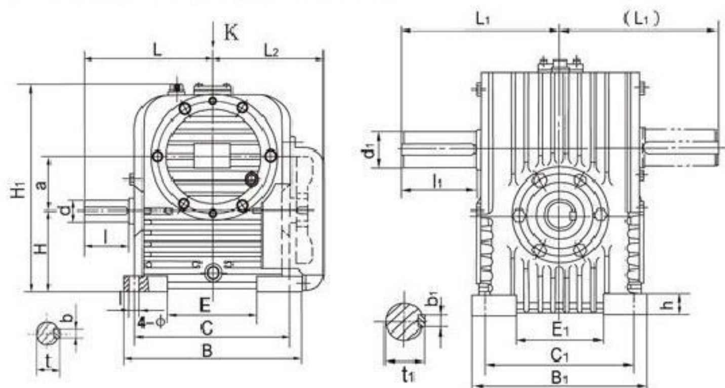
TPU型减速器（整箱式）及装配型式
