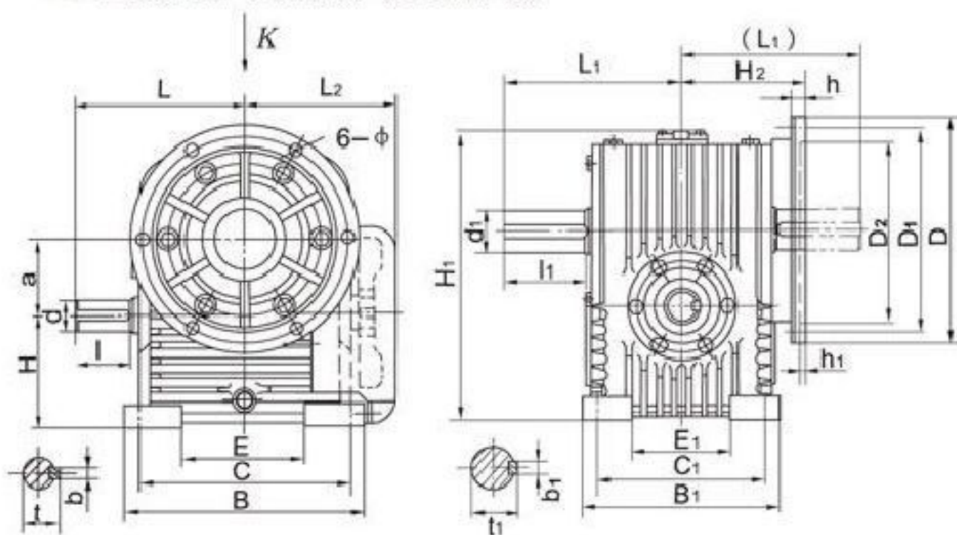
TPS型减速器（整箱式）及装配型式
