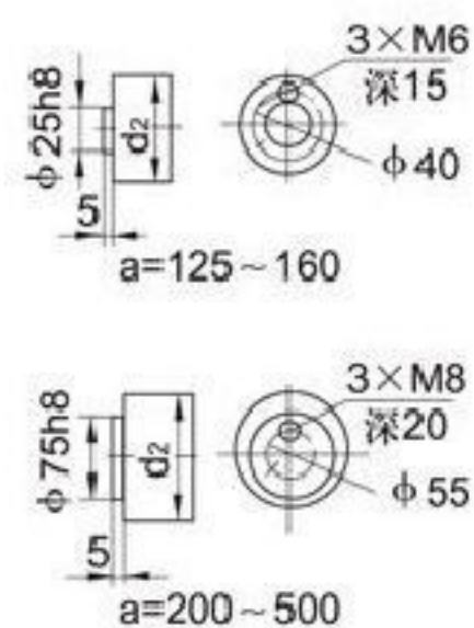
Ⅲ、ⅢF、Ⅳ、ⅣF带控制器用轴端
