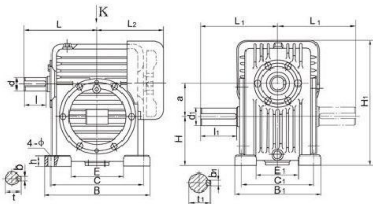
TPA型减速器（整箱式）及装配型式
