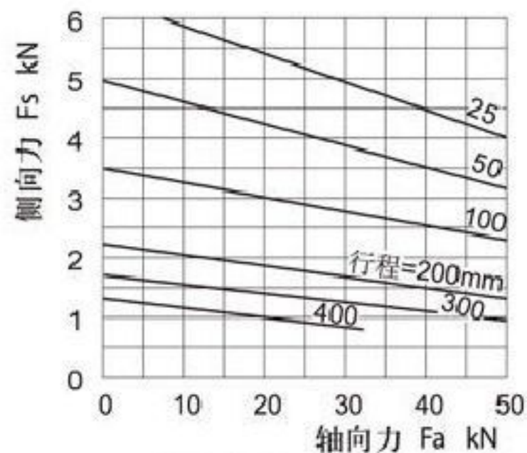
图6 SWL5(QWL5)
