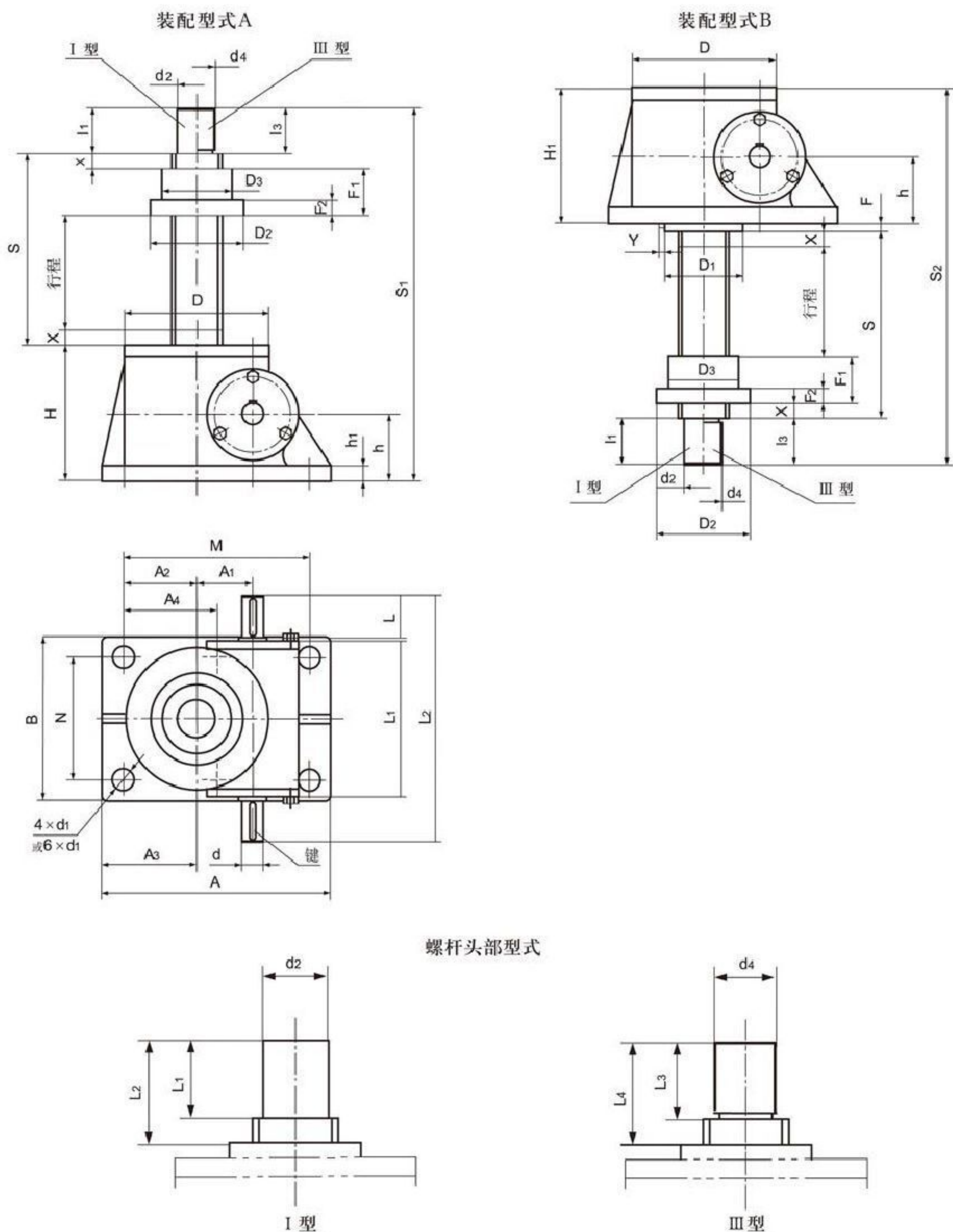
图2 2型结构型式
