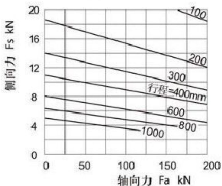
图9 SWL25(QWL25)
