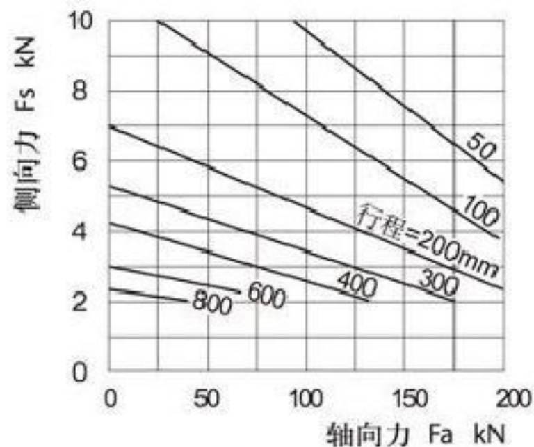
图8 SWL20(QWL20)
