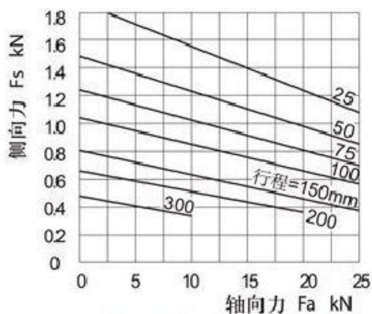
图5 SWL2.5(QWL2.5)
