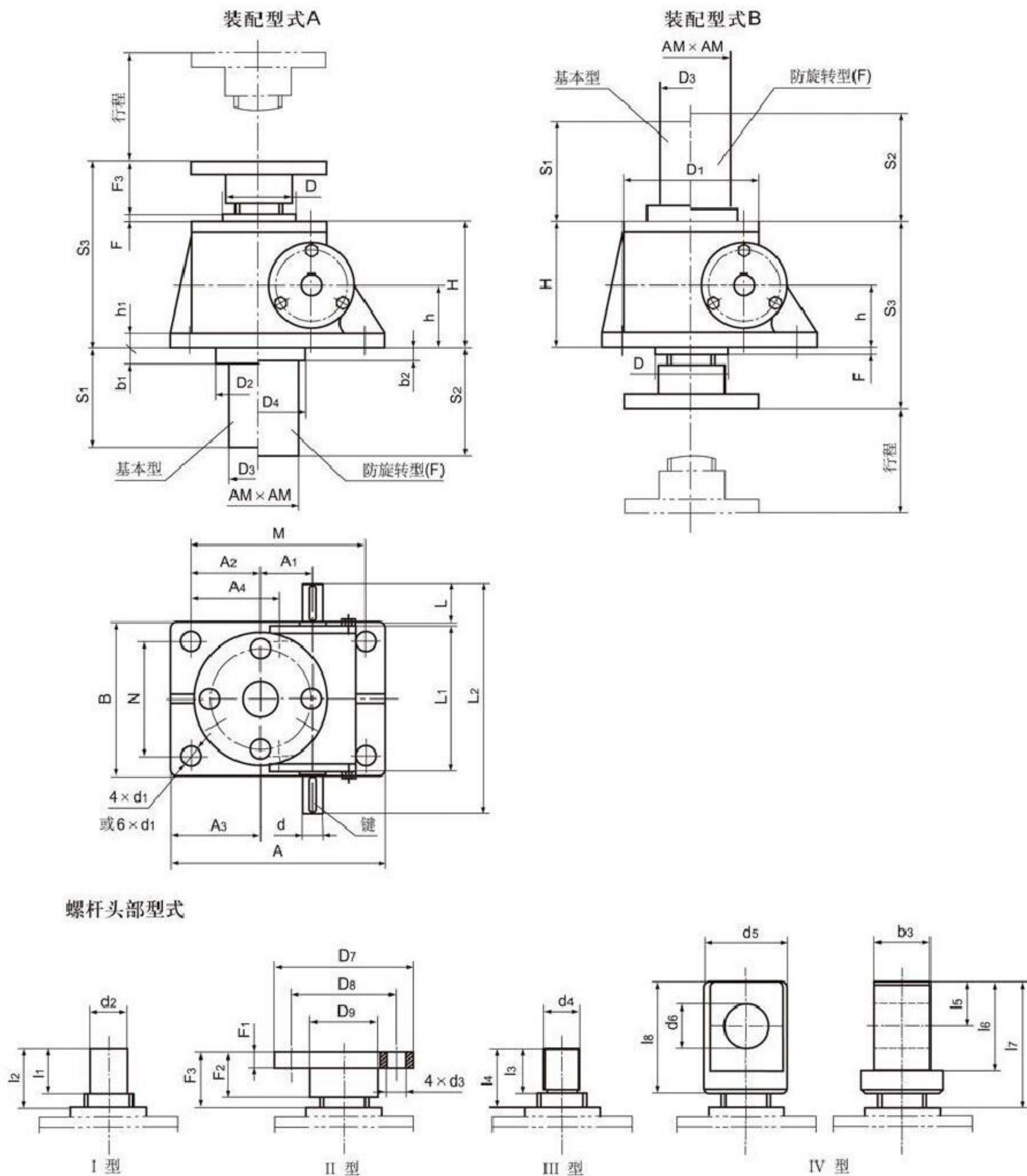
图1 1型结构形式
