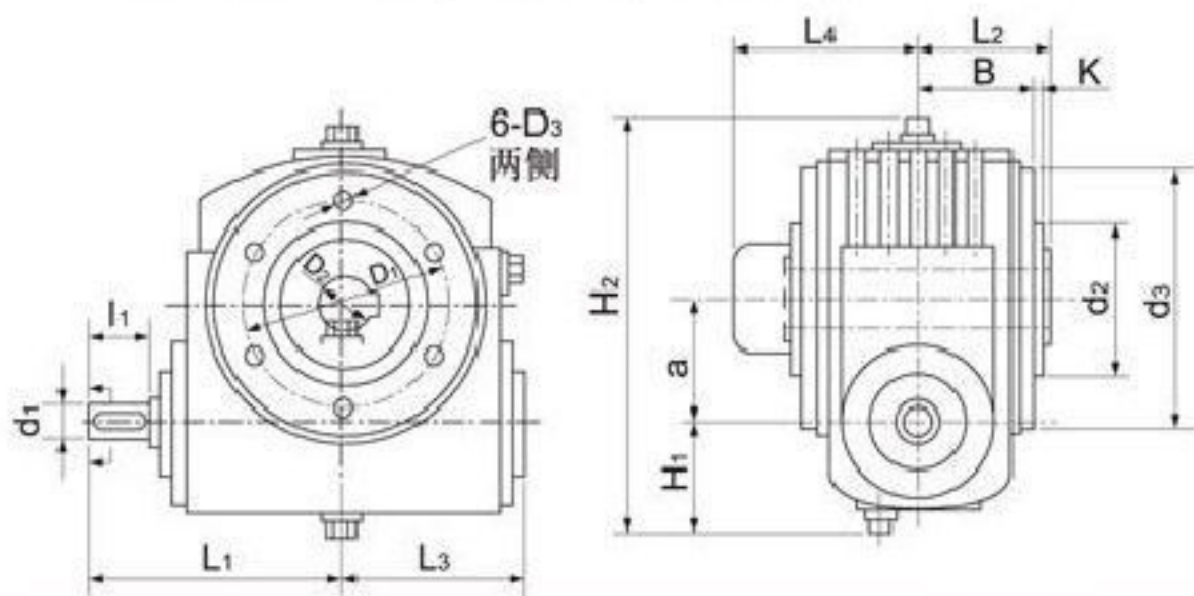
SCWU63—100型减速器外形尺寸
