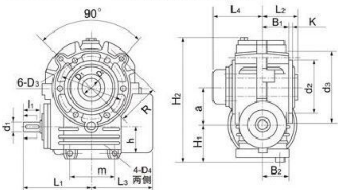
SCWU125—315型减速器外形尺寸
