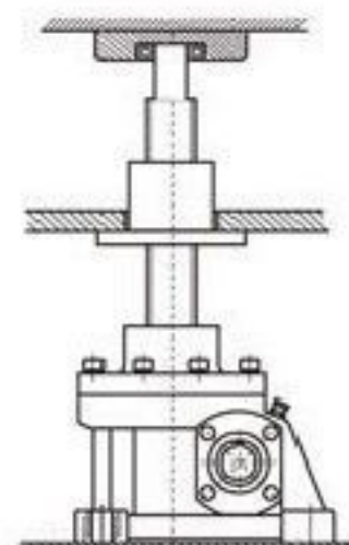
底座回定—轴端固定或支撑
