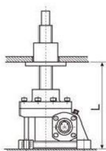
底座回定—轴端自由
