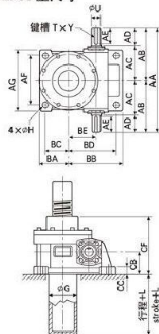
GLFSJ型尺寸
